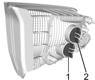
Показана сторона пассажира (вариант без светодиодных ламп)
