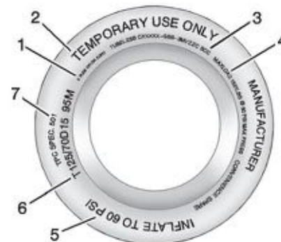
Пример маркировки шины неполноразмерного запасного колеса (1) Материал корда шины. Тип корда и количество слоев в боковине шины и под ее протектором.
